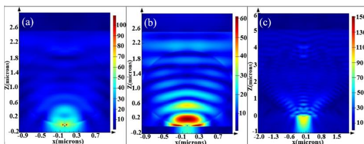
شکل ۳: (a) توزیع میدان الکتریکی در میکروکره SiO_2 به همراه نانوذرات طلا بدون زیر لایه سیلیکون، (b) با زیر لایه سیلیکون، (c) توزیع میدان الکتریکی در میکروکره SiO_2 با شعاع ۲ میکرون با نانوذرات طلا.
