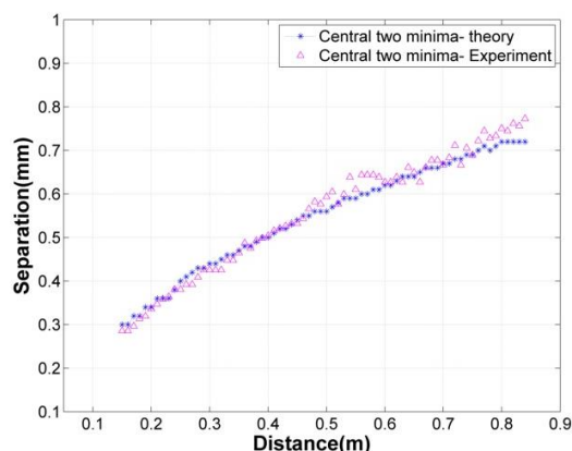
شکل ۴: فاصله‌ی بین دو کمینه مرکزی طرح پراش از نوار فازی برحسب فاصله نوار فازی از صفحه‌ی مشاهده‌ی z .
