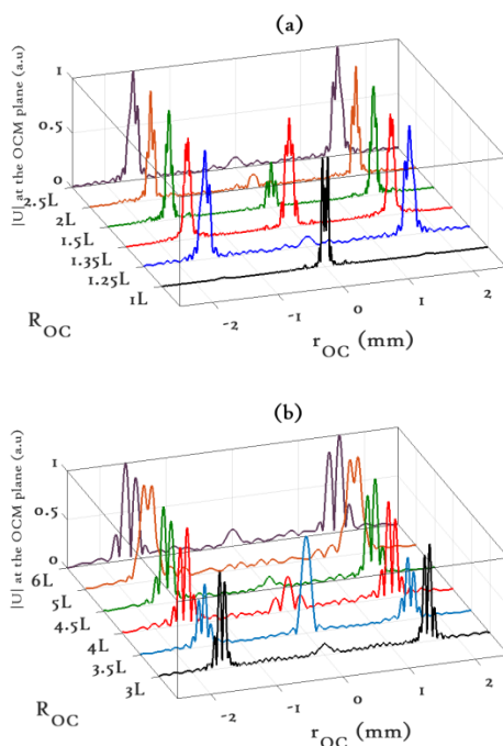
شکل ۲ پروفایل عرضی باریکه‌ی خروجی حلقوی-شکل را بر حسب تغییرات شعاع انحنای آینه‌ی خروجی (a) در بازه L تا L
