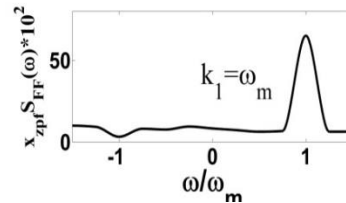
شکل ۲: طیف نویز کوانتومی نیروی اپتیک برحسب تابعی از فرکانس \omega / \omega_m
