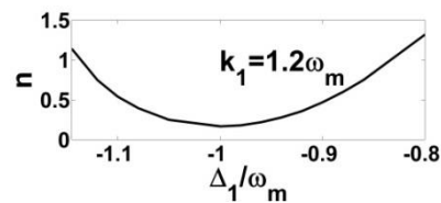
شکل ۳: در این شکل تعداد فونون ها بر حسب \Delta_1 / \omega_m نشان داده شده است در این شرایط سردسازی رخ می دهد.
