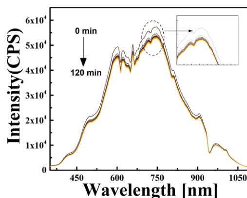
شکل ۴: طیف پایداری لامپ هالوژن تنگستن به مدت دو ساعت و ثبت هر دو دقیقه یک طیف.
