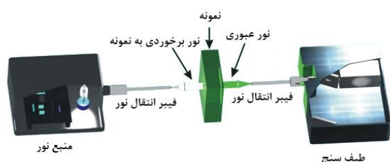
شکل ۲: شماتیک چیدمان عبوری طیف سنجی استفاده شده برای ثبت طیف‌ها.
