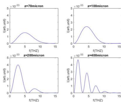
شکل ۲. توزیع فرکانسی میدان تراهرتزی در محیط غیرخطی در طول های مختلف از نانولوله کربنی
