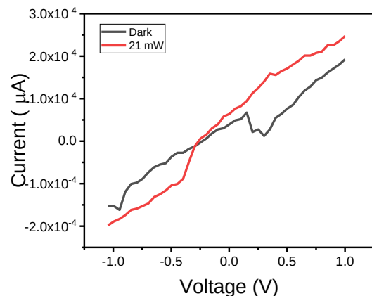
شکل ۱: نمودار جریان ولتاژ برای لایه تیتانیوم دی اکسید پرینت شده به وسیله قالب شکاف باریک در تاریکی و در معرض نور
