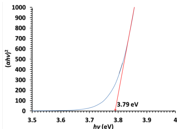
شکل ۲: نمودار (\alpha h\nu)^2 بر حسب h\nu برای اکسید ایندیوم تهیه شده در حضور گلیسین.
