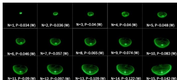
شکل ۴: طرح پراش SSMP در محلول (μg/cc) ۲۰۰ از اکسید گرافن در NMP
