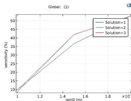
شکل شماره ۲: شبیه سازی با نرم افزار کامسول با پارامترهای ذکر شده
