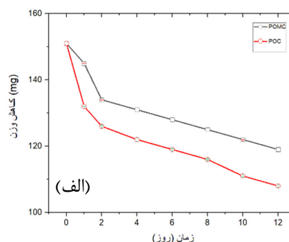
شکل ۲- (الف) نمودار تخریب پلیمرهای POMC و POC در ۱۲ روز، (ب) فیبرنوری پلیمری پیچانده شده در اطراف میله.
