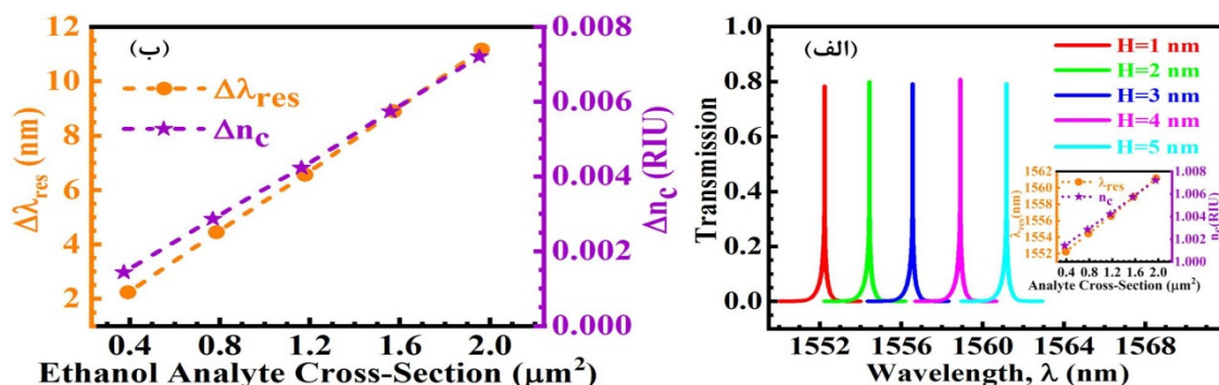
شکل ۳- الف) نمودارهای جابه‌جایی طیف عبور، ب) پوشش فیبر بلور فوتونی بهینه‌شده به اِزاء ضخامت (H) و سطوح مختلف لایه اتانول.
