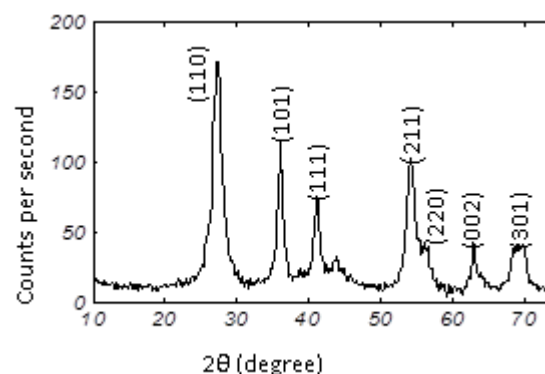
شکل ۱: طیف XRD نانوذرات تیتانیوم دی اکسید تهیه شده
