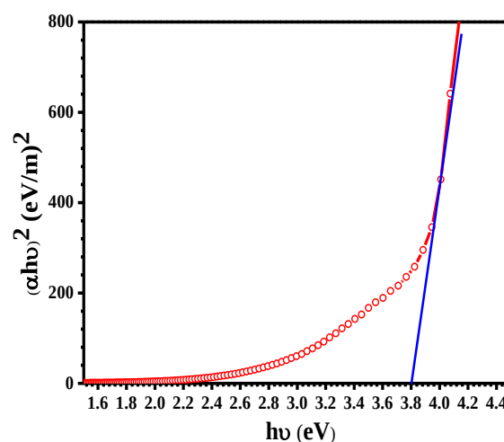
شکل ۷: نمودار (\alpha h\nu)^2 بر حسب انرژی فوتون برای لایه نازک تیتانیوم دی‌اکسید تهیه شده با روش غوطه‌وری
