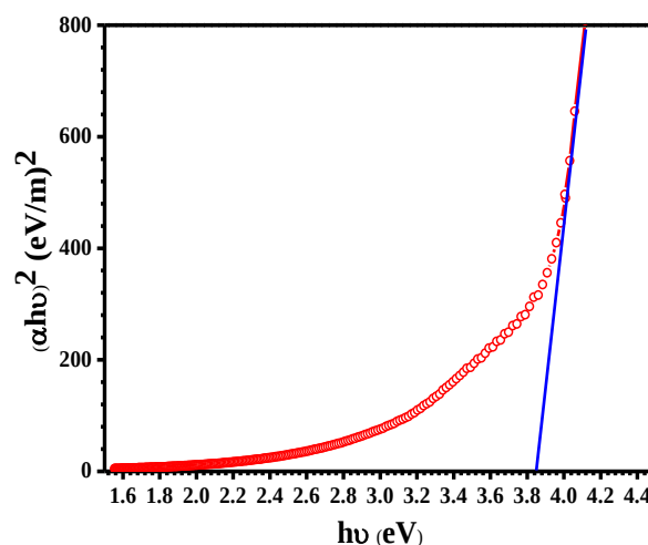
شکل ۶: نمودار (\alpha h\nu)^2 بر حسب انرژی فوتون برای لایه نازک تیتانیوم دی‌اکسید تهیه شده با روش چرخشی
