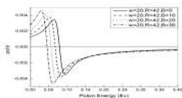
شکل ۴: تغییرات ضریب شکست کل براساس انرژی فوتون ورودی به ازای مقادیر متفاوت میدان مغناطیسی و w = 20A^0 , R = 42A^0
