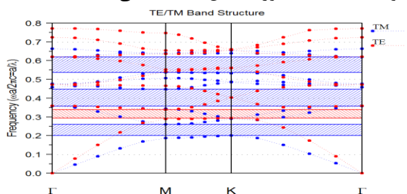
شکل ۱. ساختار باند کریستال فوتونیک مورد نظر
