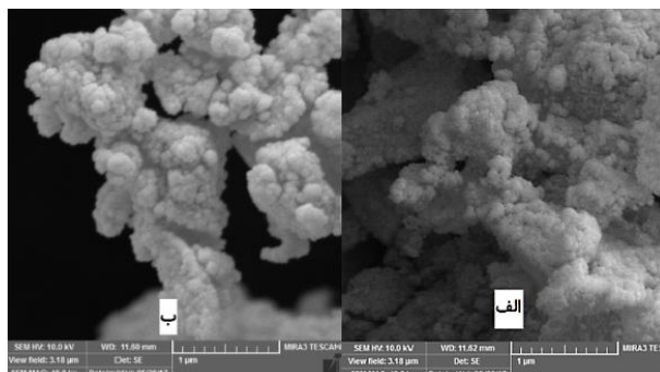
شکل ۲- الف) تصویر SEM نمونه‌ی تیتانیوم دی اکسید قبل از اعمال پلاسما ب) تصویر SEM نمونه‌ی تیتانیوم دی اکسید اصلاح شده توسط پلاسمای تخلیه تابان آرگون به مدت ۴۵ دقیقه و فشار ۰/۳ تور
