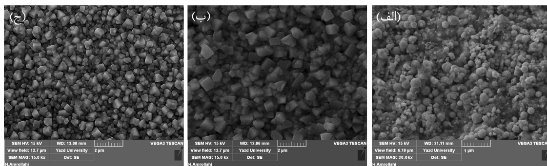
شکل ۱- تصویر SEM (الف) چارچوب آلی-فلزی (Al) MIL53 سنتز شده روش حلال گرمایی، (ب) سطح پروسکایت پایه با زیرلایه \text{TiO}_2 (ج) سطح پروسکایت با زیرلایه \text{TiO}_2/\text{MIL53}(\text{Al})
