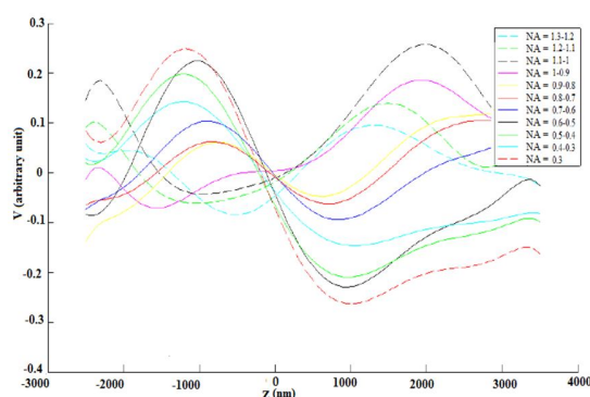
شکل ۳- نمودارهای مربوط به تفاضل ولتاژ دو گشودگی عددی متوالی عدسی چگالنده برحسب جابه‌جایی محوری ذره‌ی ۱/۰۱ میکرونی.
