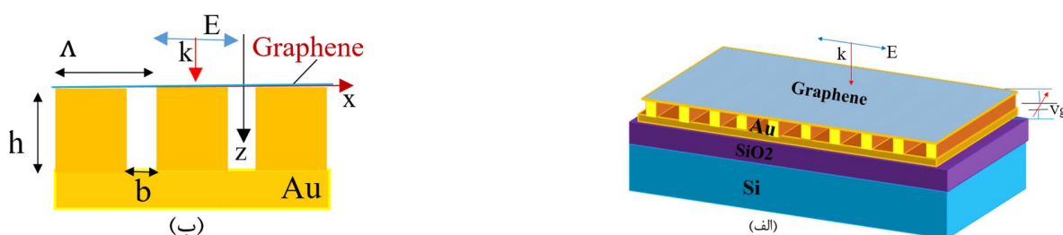
شکل ۱: (الف) نمای سه بعدی از آشکارساز نوری مبتنی بر گرافن، (ب) نمای برش دو بعدی از نانو توری و گرافن.
