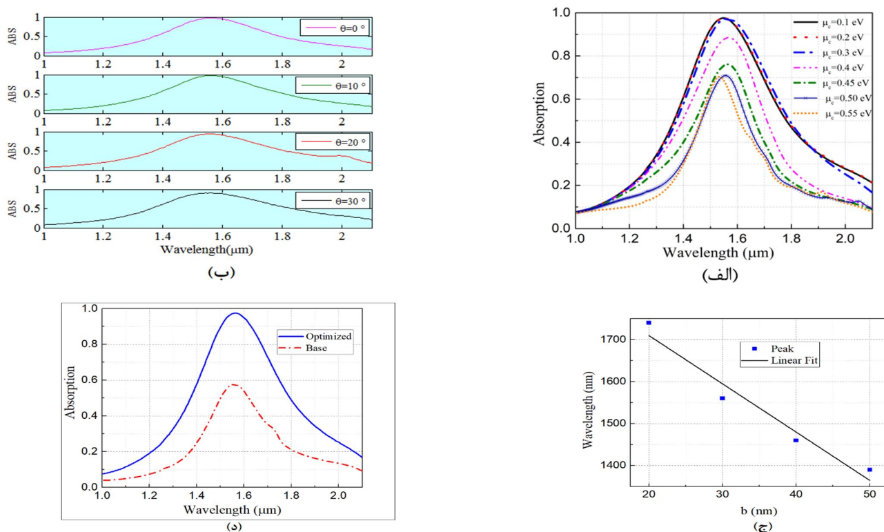
شکل ۲- (الف) طیف جذب ساختار به ازای پتانسیل‌های شیمیایی مختلف، (ب) طیف جذب ساختار به ازای زوایای مختلف منبع نور تابشی، (ج) طول موج پیک جذب به ازای عرض شیارهای مختلف نانو توری، (د) طیف جذب ساختار بهینه شامل توری پراش با گرافن و ساختار پایه شامل توری پراش بدون گرافن.
