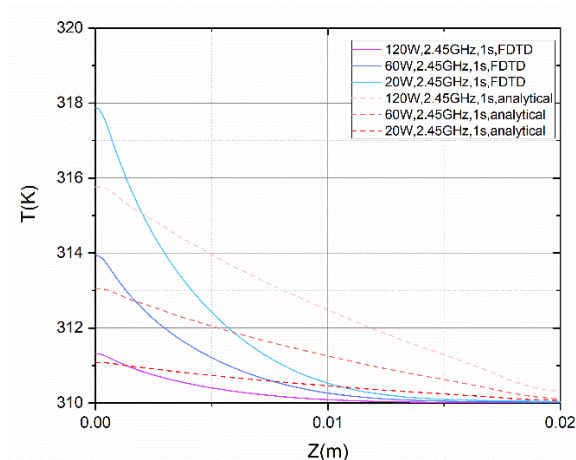
شکل ۱: مقایسه حل تحلیلی و عددی برای توان های مختلف در فرکانس ۲.۴ گیگاهرتز. در نمودار، خطوط پیوسته جواب عددی و خطوط گسسته پاسخ تحلیلی را نشان می دهند.
