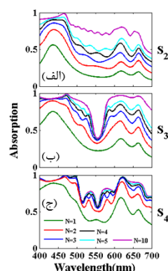
شکل ۴: اثر N بر روی جذب S2, S3 و S4 در ساختار III.
