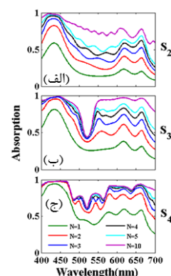
شکل ۳: اثر N بر روی جذب S2, S3 و S4 در ساختار II.
