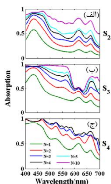
شکل ۲: اثر دوره‌ی تناوب بر روی جذب S_2 ، S_3 و S_4 در ساختار I.
