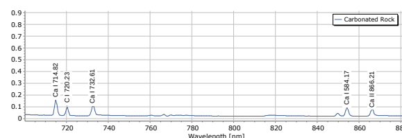
شکل ۹ ناحیه فروسرخ طیف سنگ کربناته در محدوده ۸۸۰ nm - ۷۰۰ nm
