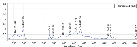
شکل ۸ ناحیه مرئی طیف سنگ کربناته در محدوده ۶۸۰ nm - ۵۴۰ nm
