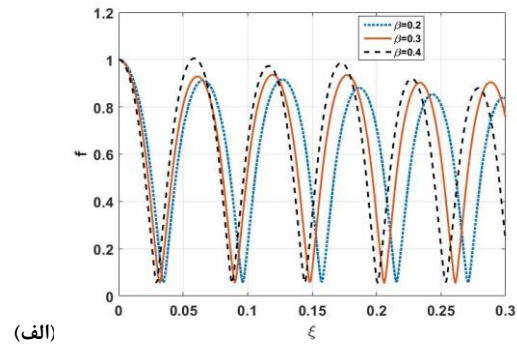
(الف) شکل ۲: تغییرات شعاع لکه لیزر بر در راستای انتشار، برای چگالی الکترونی با (الف) پروفایل نمایی و (ب) پروفایل خطی
