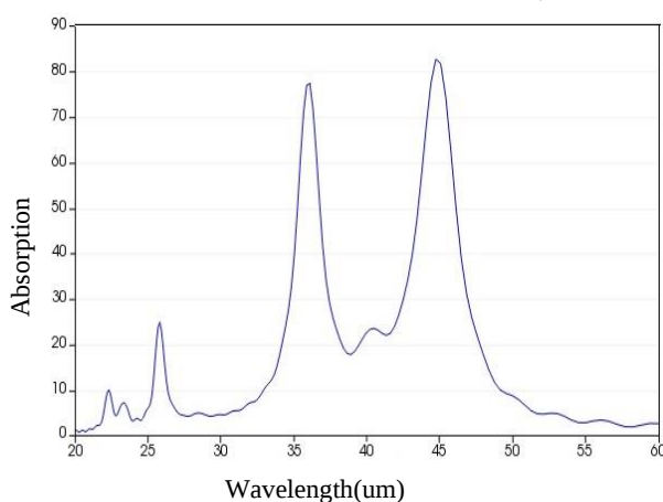
شکل ۲: طیف جذبی ساختار شکل ۱- (ب) که در طول موج های \lambda = 44/7 \mu m و \lambda = 35/846 \mu m دو قله جذبی ۸۰٪ مشاهده می‌شود.
