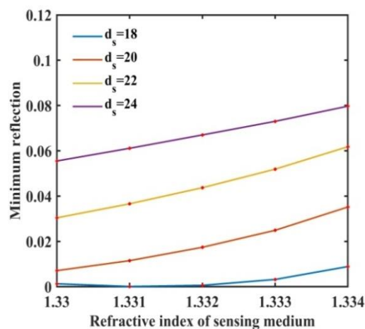
شکل ۵ حساسیت تصویربرداری در ضخامت‌های متفاوت لایه میانی
