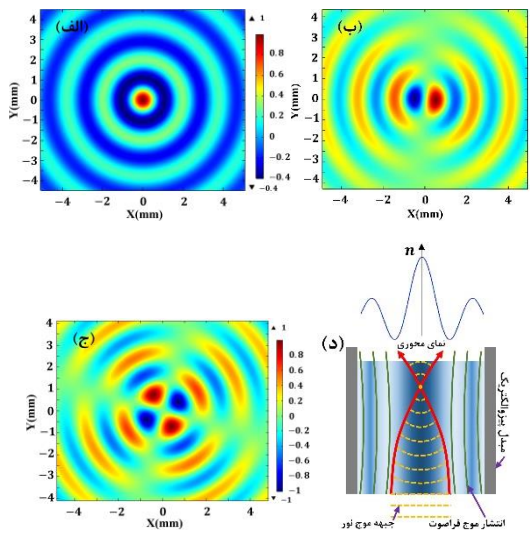
شکل ۳: الگوهای تداخل فضایی تولید شده در فانتوم بافت مغز توسط موج فشاری فراصوت. به ازای ولتاژ ورودی ۳۴ v (الف) مد پایه ( m = 0 ) در فرکانس ۸۲۸،۶۴ kHz (ب) مد مرتبه دوم ( m = 1 ) در فرکانس ۸۴۸،۰۵ kHz (ج) مد مرتبه سوم ( m = 2 ) در فرکانس ۸۶۷،۲۸ kHz (د) شماتیک مدولاسیون ضریب شکست و هدایت نور درون فانتوم با تشکیل امواج ایستاده فراصوت.
