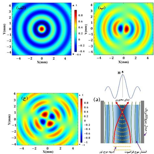
شکل ۳: الگوهای تداخل فضاوی تولید شده در فانتوم بافت مغز توسط موج فشاری فراصوت. به ازای ولتاژ ورودی ۳۴ v (الف) مد پایه ( m=0 ) در فرکانس ۸۶۷،۲۸ kHz، (ب) مد مرتبه دوم ( m=1 ) در فرکانس ۸۴۸،۰۵ kHz و (ج) مد مرتبه سوم ( m=2 ) در فرکانس ۸۲۸،۶۴ kHz تشکیل شده‌اند. (د) شماتیک مدولاسیون ضریب شکست و هدایت نور درون فانتوم با تشکیل امواج ایستاده فراصوت.
