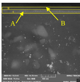
شکل ۲. تصویر FESEM از مقطع نمونه زرین فام. مکان A و B تعیین شده در شکل، به ترتیب بیانگر تشکیل نانوذرات نقره در بستر لعاب و ایجاد یک لایه دی‌الکتریک روی سطح نمونه می‌باشند.
