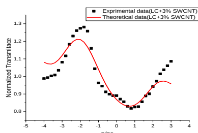
شکل ۶: نمودار روبش z با دریچه بسته برای سل بلورمایع + ۳٪ نانولوله کربن
