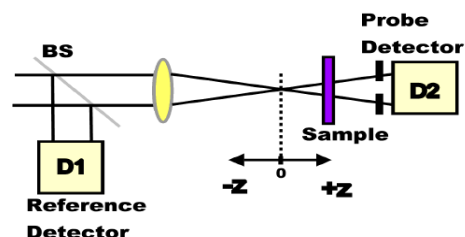
شکل ۲: طرح شماتیک روبش z با دریچه بسته [۱۰]
