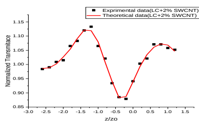
شکل ۵: نمودار روبش z با دریچه بسته برای سل بلورمایع + ۲٪ نانولوله کربن
