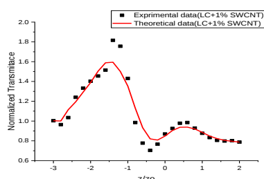
شکل ۴: نمودار روبش z با دریچه بسته برای سل بلور مایع + ۱٪ نانولوله کربن
