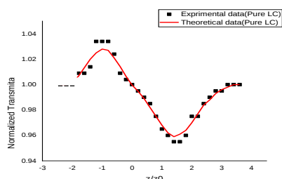
شکل ۳: نمودار روبش z با دریچه بسته برای سل بلورمایع خالص
