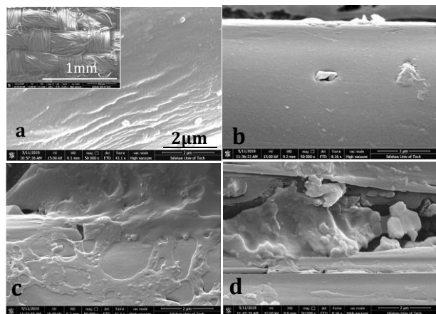
شکل ۴: تصاویر مربوط به میکروسکوپ الکترونی (SEM) بر روی زیرلایه‌ی پارچه پلی استر (a): قبل از لایه‌های نشانی اکسید مولیبدن، (b) الی (d): پس از لایه‌های نشانی به ترتیب برای نمونه‌های S1 الی S3
