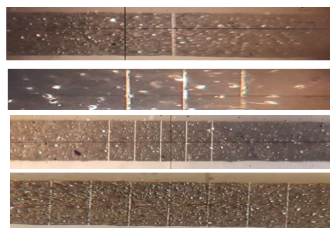
شکل ۲: نمایش میکروسکوپی خطوط لیزر بر روی نوارهای مغناطیسی، یک، سه، پنج و هفت شیار
