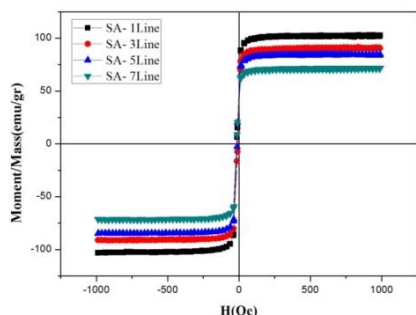
شکل ۳: نمایش منحنی مغناطش نوار مغناطیسی تحت تاثیر تابش نور لیزر اگزایمر با شیارهای متفاوت
