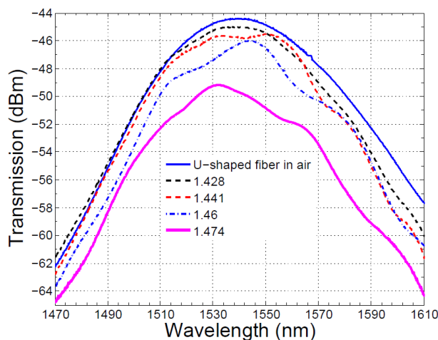
شکل ۳. طیف عبوری از حسگر به ازای تغییرات ضریب شکست محیط اطراف.
