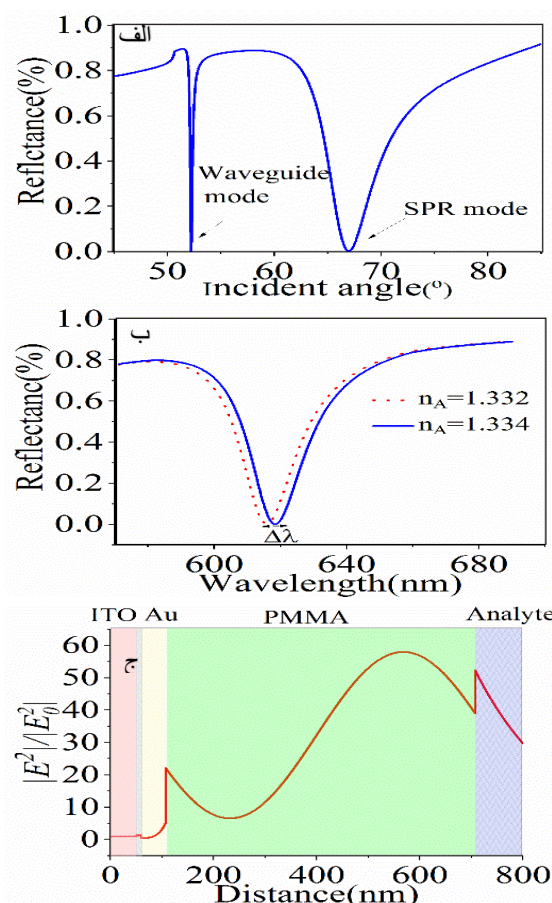
شکل ۲. الف) نمودار بازتاب بر حسب زاویه تابش و ب) طول موج. ج) پروفایل میدان الکتریکی در لایه‌های مختلف حسگر
