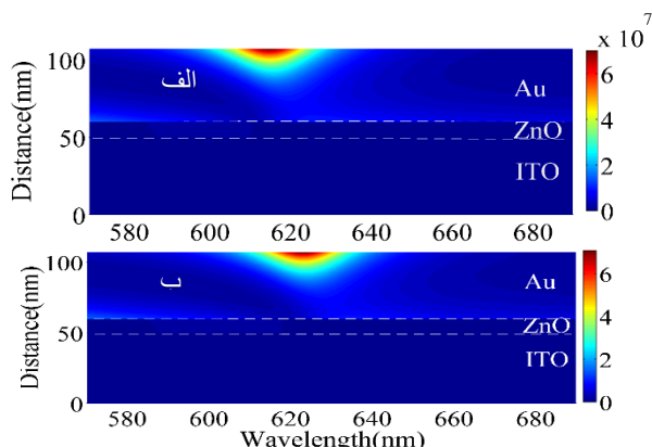
شکل ۳. پروفایل جذب در لایه‌های مختلف TCO-I-M برای طول‌موج‌های مختلف. الف) برای ضریب شکست آنالیت ۱/۳۳۲ و ب) ۱/۳۳۸
