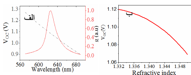
شکل ۴. الف) ولتاژ مدار باز و رسانایی ITO-I-M برای طول موج‌های مختلف. ب) پاسخ الکتریکی حسگر برای ضریب شکست‌های مختلف آنالیت
