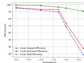
شکل ۵: نمودارهای تغییرات بازده غلاف برحسب تغییرات ضریب میرایی در فرکانس ثابت ۳ تراهرتز و ضخامت غلاف ۱۳۳ میکرومتر. نمودار قرمز رنگ برای بازدهی رو به جلو و نمودار سبز رنگ برای بازدهی رو به عقب را معین می‌کنند.
