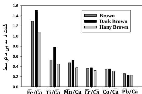
شکل ۳: نمودار کالیبراسیون ستونی نسبی شدت های متوسط
