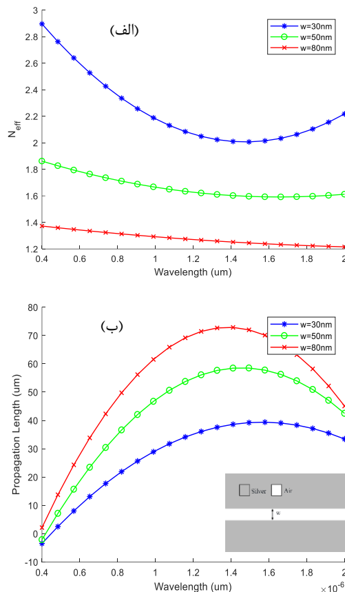
شکل ۱: (الف) بخش حقیقی ضریب شکست موثر (ب) طول انتشار، به عنوان تابعی از طول موج برای عرض های مختلف.
