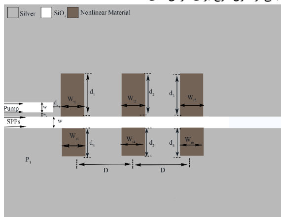
شکل ۲: طرحواره موجبر پلاسمونیک چند دندانان ای با توجه به شکل ۱ (ب)، با افزایش عرض دندانان ها بخش حقیقی ضریب شکست موثر کاهش و طول انتشار افزایش می یابد. شکل ۲ طرحواره ساختار سویچ تمام نوری را نشان می دهد که دارای موجبر با ساختار چند دندانان ای و دو لایه فلزی در کنارها است. فلز مورد استفاده، نقره است که گذردهی نسبی آن را می توان با مدل درود به صورت زیر توصیف کرد:
