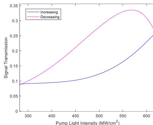
شکل ۵: میزان عبور با افزایش و کاهش شدت پمپ ورودی (حالت دوپایداری)
