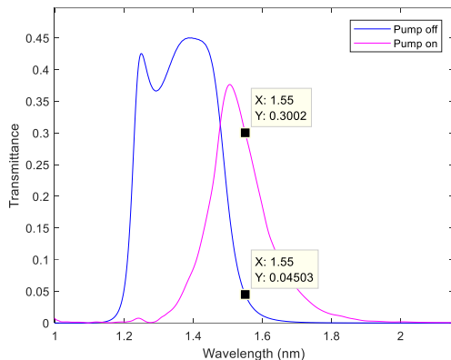
شکل ۴: عبور سیگنال زمانی که پمپ در حالت خاموش و روشن قرار دارد. طول موج پمپ ۱ میکرومتر و طول موج سیگنال ۱.۵۵ میکرومتر می باشد. شدت پمپ برابر است با 650MW/cm^2
