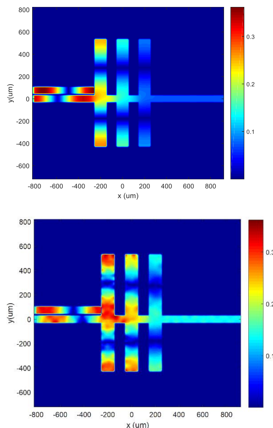
شکل ۶: توزیع میدان مغناطیسی زمانی که پمپ در حالت الف) خاموش و ب) روشن می باشد.
