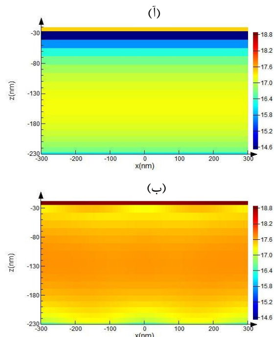
شکل (۵)- نمودار سه بعدی جذب در صفحه XZ برای آ (بدون نانوذره ب) آرایه ای از نانوذرات با ارتفاع ۱۲۰ nm، قطر ۱۰۰ nm و دوره تناوب ۱۳۰ nm در فاصله ۱۰۰ nm از آرایه.
