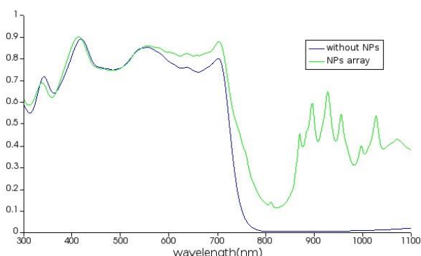
شکل (۴)- نمودار جذب برای حالت بدون نانوذره و حالت آرایه ای از نانومیله های نقره.
