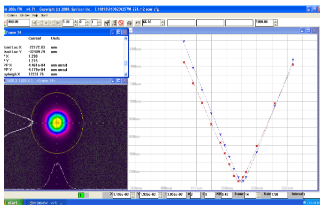
شکل ۵: کیفیت باریکه لیزر در توان 3/02 کیلووات.
