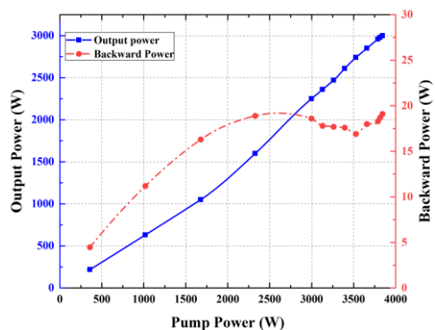
شکل ۴: نمودار توان نور برگشتی (رنگ قرمز) و توان خروجی (رنگ آبی) بر حسب توان پمپ شده در حالت پمپاژ از دو طرف. با توجه به شکل آستانه ناپایداری مدی در چیدمان پمپاژ از دو طرف در مقایسه با چیدمان پمپاژ از انتها و روبرو بالاتر است.
