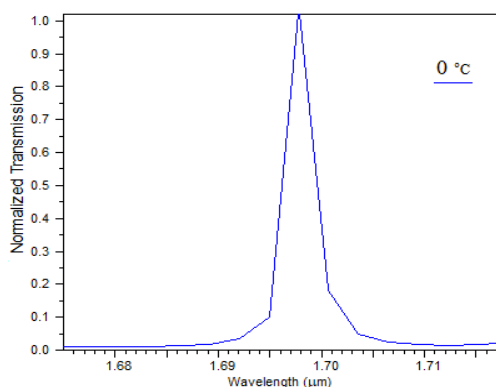
شکل (۳): طیف نرمالیزه شده خروجی نانو حسگر بدون اعمال دما.
