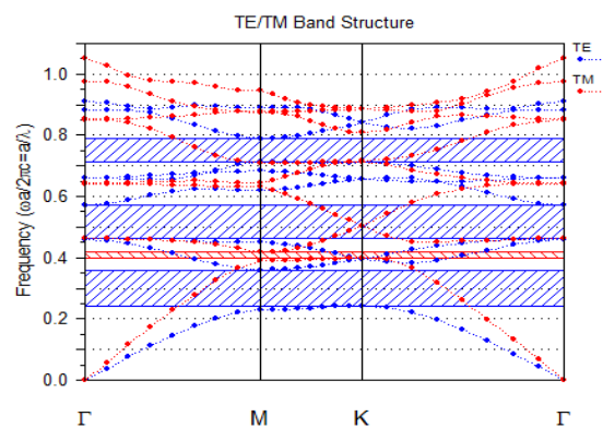
شکل (۲): نمودار شکاف باند فوتونی نانو حسگر دما فوتونیک کریستالی.
