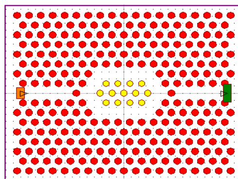
شکل (۱): ساختار نانو حسگر دما فوتونیک کریستالی.
