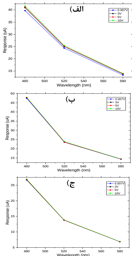
شکل ۵. پاسخ فوتودیودها به تابش نور. الف) SGPD30C، ب) BPW34B، ج) BS500B
