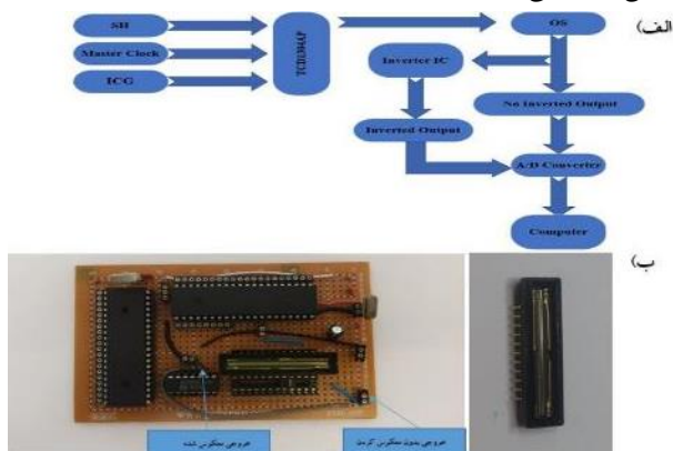
شکل ۱. الف: بلوک دیاگرام مداری. ب: برد طراحی شده برای راه‌اندازی CCD به همراه تصویر TCD1304AP
