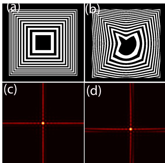
شکل ۱: در ردیف بالا به ترتیب دو تیغه‌ی فرنل شبیه سازی شده محوری و برون محوری و در ردیف پایین نیز توزیع شدت متناظر هر دو تیغه مربوطه در شکل‌های پایینی نشان داده شده‌است.
