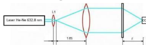
شکل ۴: چیدمان آزمایشگاهی
