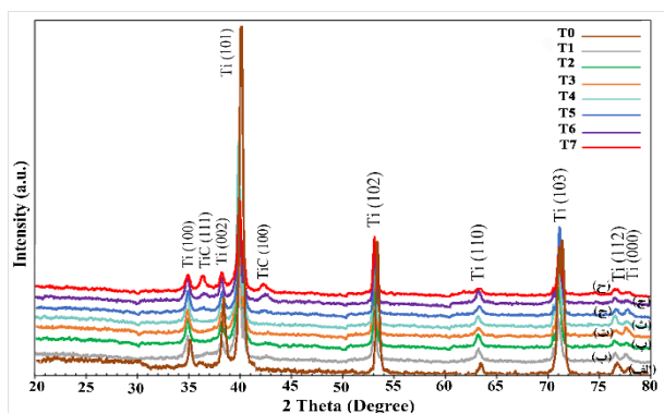
شکل ۱: الگوی پراش پرتو ایکس (الف) T۰، (ب) T۱، (پ) T۲، (ت) T۳، (ث) T۴، (ج) T۵، (چ) T۶، (ح) T۷.
