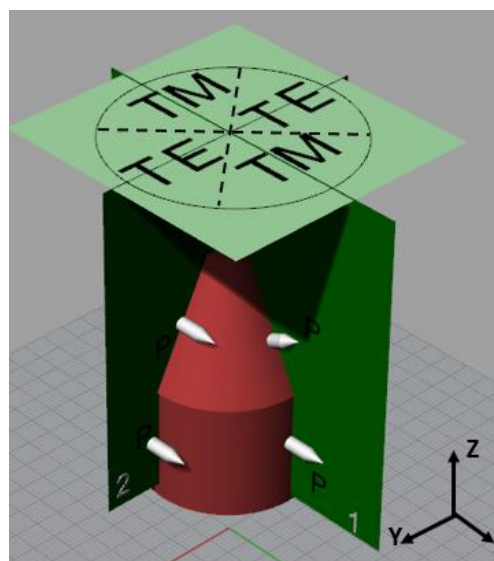
شکل ۳: تحول قطبش در عدسی شیئی. P جهت قطبش نور را نشان می دهد
