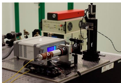
شکل ۱: چیدمان آزمایشگاهی مربوط به میکروماشین‌کاری Yb:YAG - a: لیزر پمپاژ دیودی b: میکرولیزر کیوسویچ انفعالی Nd:YAG - c: بیم اکسپندر d: لنز اف تا e: ماده هدف (Yb:YAG) f: استیج میکرومتری
