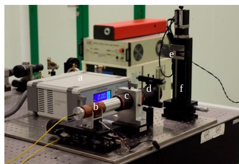
شکل ۱: چیدمان آزمایشگاهی مربوط به میکروماشین‌کاری Yb:YAG - a: لیزر پمپاژ دیودی b: میکرولیزر کیوسویچ انفعالی Nd:YAG - c: بیم اکسپندر d: لنز اف تتا e: ماده هدف (Yb:YAG) f: استیج میکرومتری
