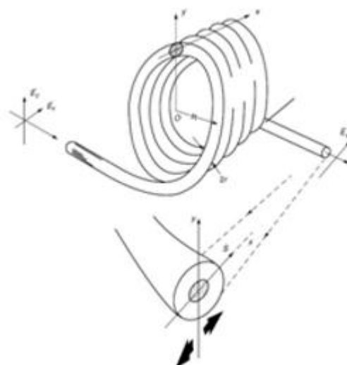
شکل ۶: فیبرنوری حلقه شده برای ساخت صفحه های موج.
