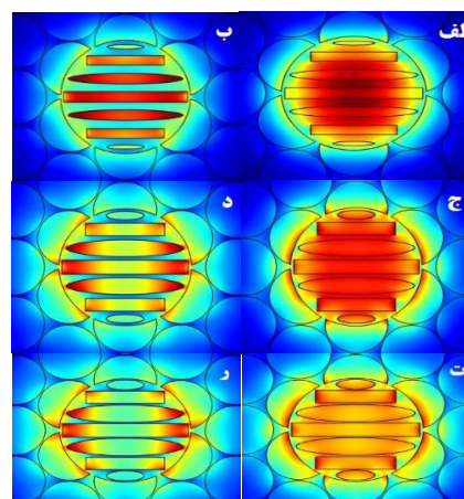
شکل ۳: توزیع شدت در (الف) تخلخل ۰.۶۳/قطبش x، (ب) تخلخل ۰.۶۳/قطبش y، (ج) تخلخل ۰.۷۳/قطبش x، (د) تخلخل ۰.۷۳/قطبش y (تخلخل ۰.۸۳/قطبش x، (ر) تخلخل ۰.۸۳/قطبش y (فرکانس کاری ۰.۸ تراهرتز)
