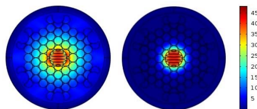
شکل ۲: توزیع شدت برای فرکانس‌های مختلف (شکل سمت راست فرکانس ۰.۸ تراهرتز و شکل سمت چپ ۰.۲ تراهرتز)
