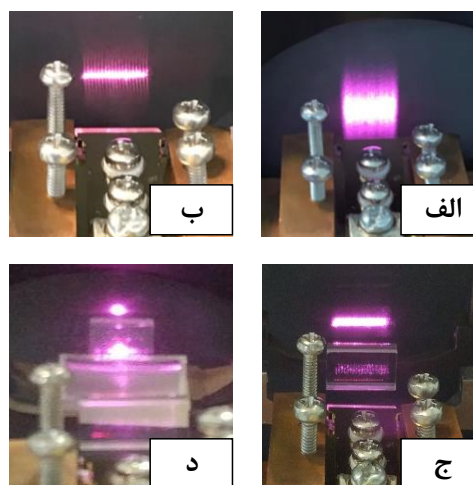
شکل ۷: پروفایل باریکه بعد از، الف: لیزر، ب: المان BTS، ج: المان SAC، د: المان تزویدگر
